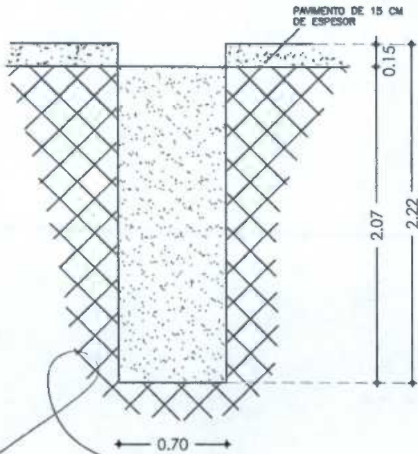
POZO PV5 ESCALA 3/4"=1' COTAS EN M.
