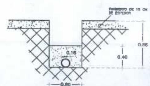
CORTE 16 ESCALA 5/8 COTAS EN M.
