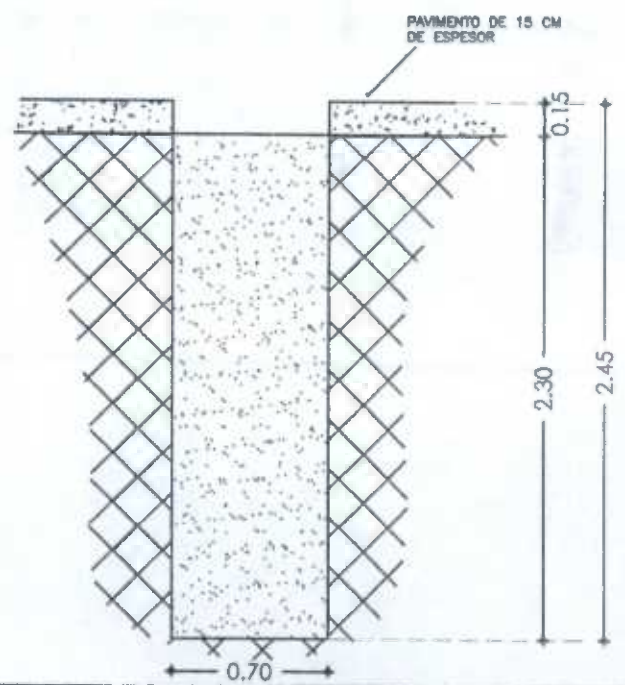
POZO PV4 ESCALA 5/E COTAS EN M.
