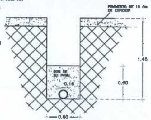
CORTE 11 ESCALA 5/8 COTAS EN M.
