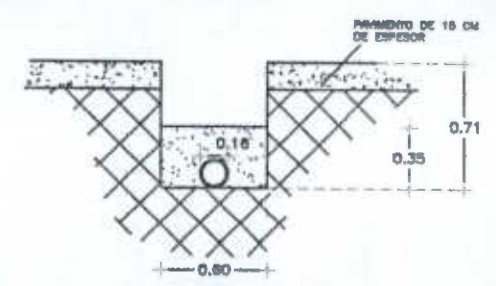
CORTE 12 ESCALA 5/8 COTAS EN M.
