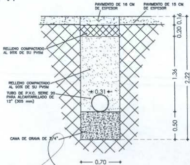
POZO PV5 ESCALA 5/E COTAS EN M.
