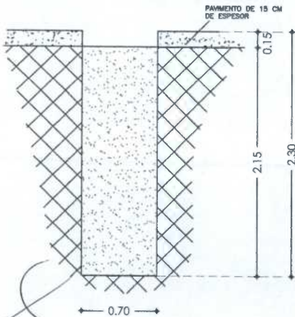
POZO PV5 ESCALA 5/E COTAS EN M.
