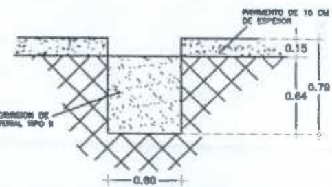
CORTE 12 ESCALA 5/E COTAS EN M.
