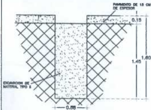
CORTE 9 ESCALA 5/E COTAS EN M.
