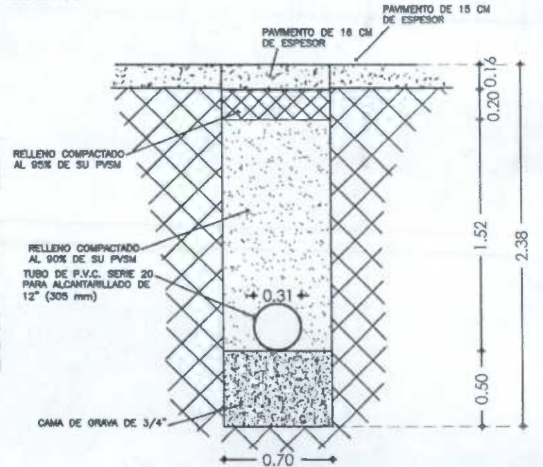
POZO PV4 ESCALA 5/E COTAS EN M.
