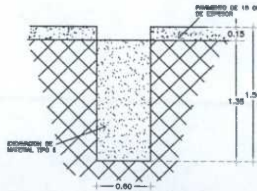
CORTE 11 ESCALA 5/E COTAS EN M.
