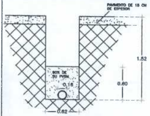
CORTE 9 ESCALA 5/8 COTAS EN M.
