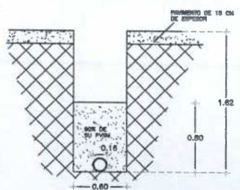
CORTE 15 ESCALA 5/8 COTAS EN M.
