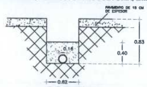
CORTE 10 ESCALA 5/8 COTAS EN M.
