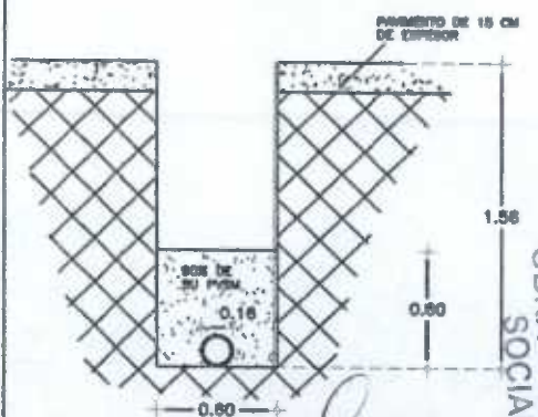
CORTE 13 ESCALA 5/8 COTAS EN M.
