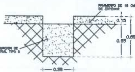
CORTE 10 ESCALA 5/E COTAS EN M.
