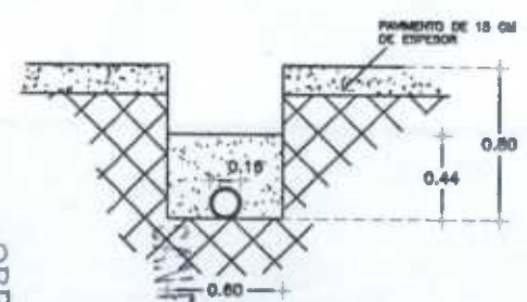
CORTE 14 ESCALA 5/8 COTAS EN M.
