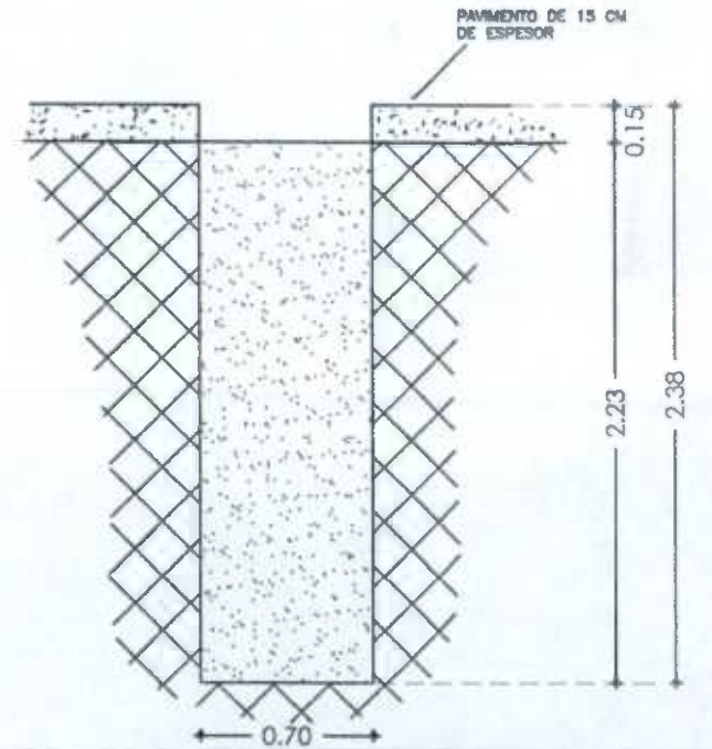
POZO PV4 ESCALA 3/4"=1' COTAS EN M.
