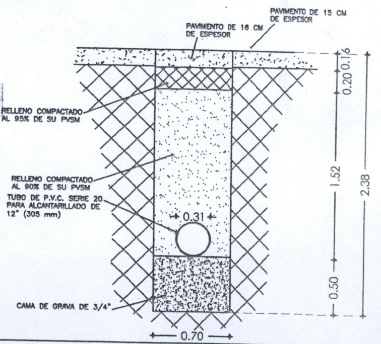
POZO PV4 ESCALA S/E COTAS EN M.
