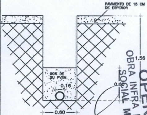
CORTE 13 ESCALA S/E COTAS EN M.
