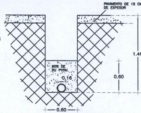
CORTE 11 ESCALA S/E COTAS EN M.
