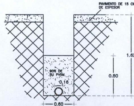
CORTE 15 ESCALA S/E COTAS EN M.
