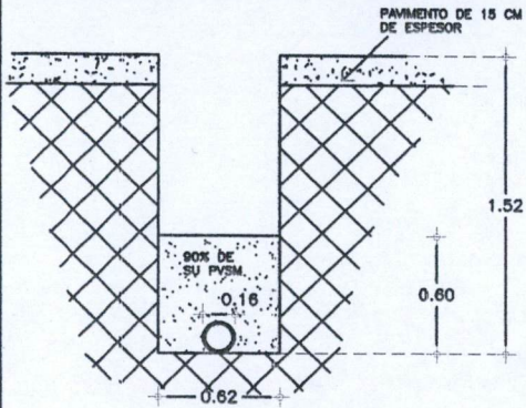
CORTE 9 ESCALA S/E COTAS EN M.
